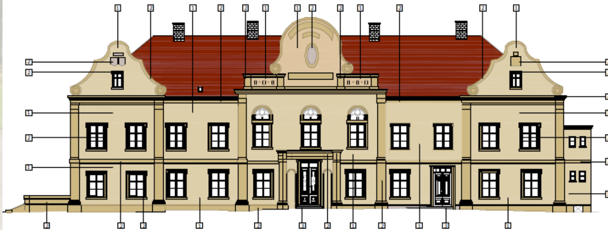
ELEWACJA PÓŁDNIOWO - WSCHODNIA STAN PROJEKTOWANY
