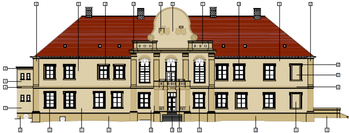
ELEWACJA PÓŁNOGNO-ZACHODNIA STAN PROJEKTOWANY
