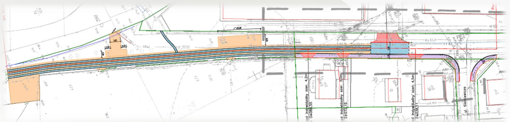
Rysunek: Wyciąg z dokumentacji projektowej zadania
