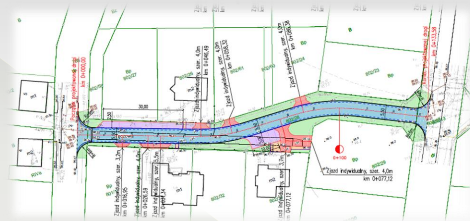
Rysunek: Wyciąg z dokumentacji projektowej zadania
