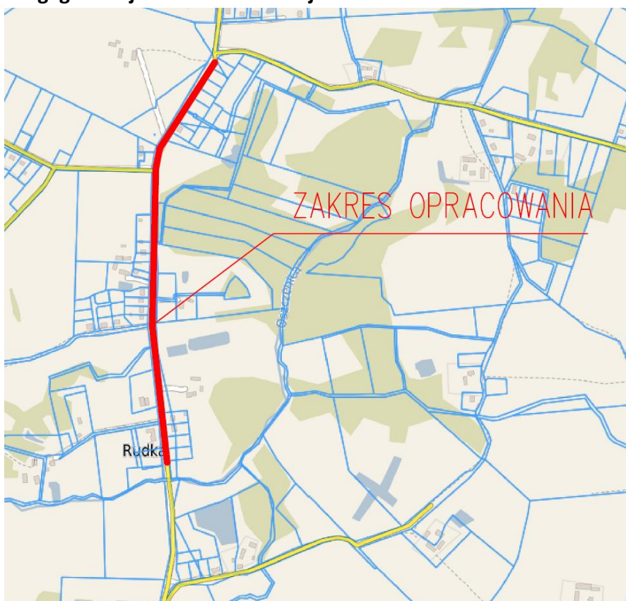
Rys. nr 13 Zakres dokumentacji zadania pn. Remont drogi gminnej nr 266512P w miejscowości Rudka
